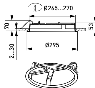
AVL21 рамка для встраиваемого монтажа
