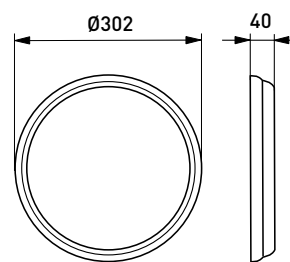
AVL28 декоративная рамка
